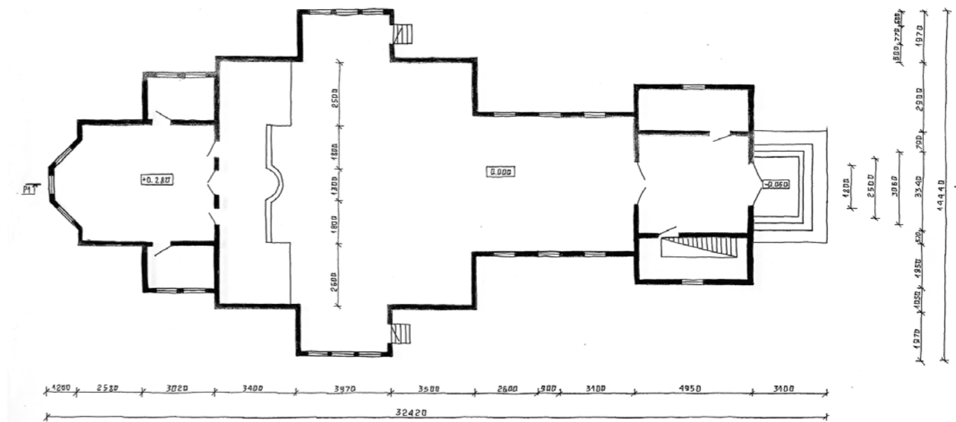
План. Обмірні креслення М. Полюхович. НУВГП. 2021
