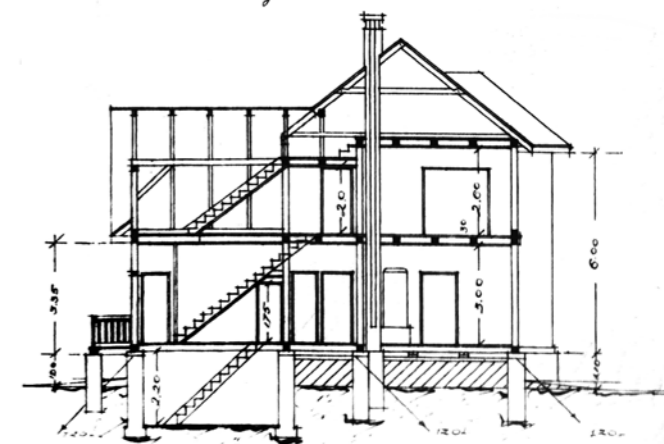
PRZEKROJ A-B
