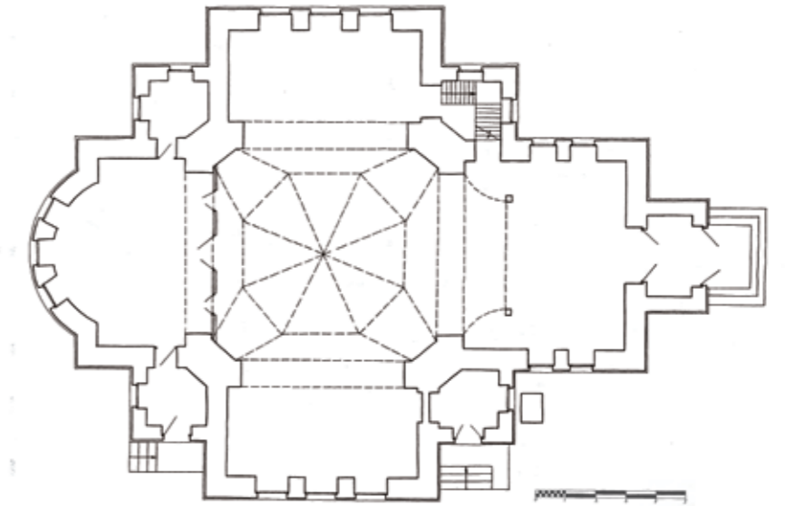
План церкви Різдва Пресвятої Богородиці. Обмірні креслення М. Лустюк. НУВГП. 2021
