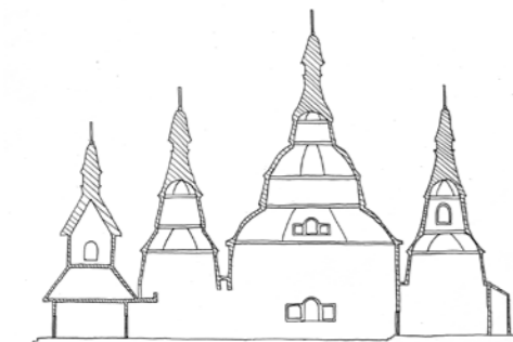
Схематичний розріз церкви. Арх. С. Тимошенко. Креслення П. Шокрути. НУВГП. 2021
