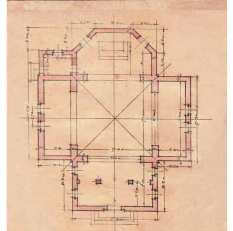
1921, Львів. Проект фасаду і плану церкви на Левандівці. Арх. С. Тимошенко. Архів церкви Св. ап. Андрія і св. Йосафата
