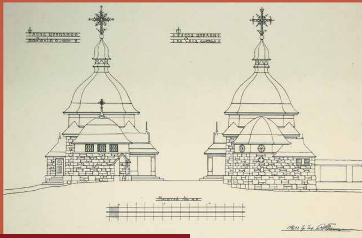
1922. Проект східного і західного фасадів церкви монастиря в Зарварниці. НМЛ, 23570
