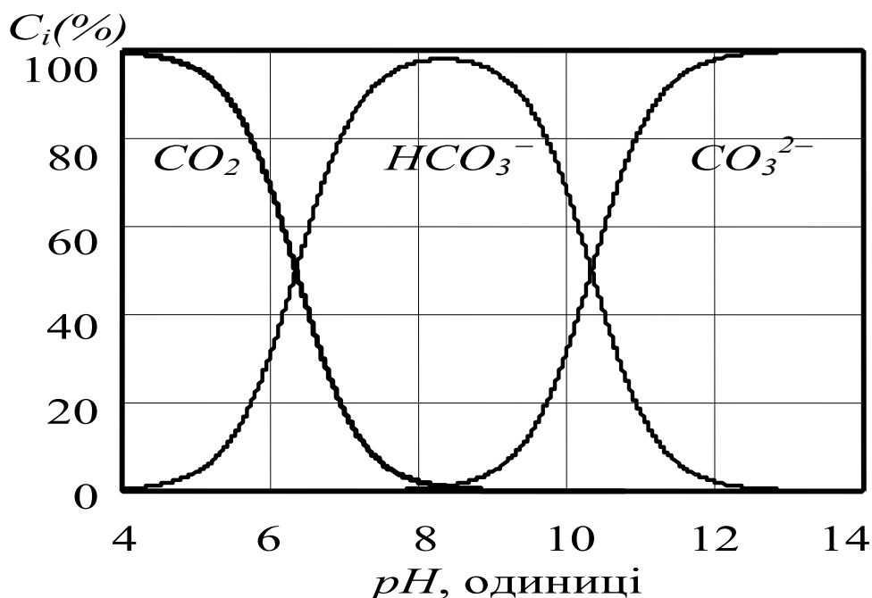
Рисунок. Відносний вміст CO_2 , HCO_3^- та CO_3^{2-} в залежності від pH
